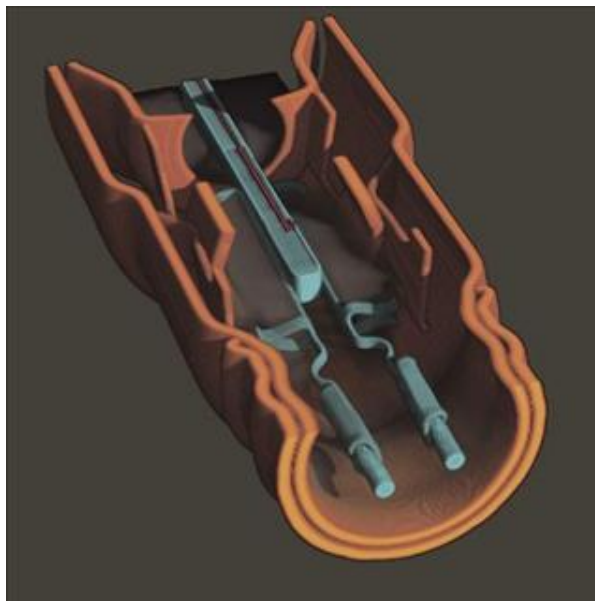
Elektronisk connector-stik. Tværsnit gennem CT-scanning gør det muligt at inspicere indvendige geometrier og komponenter.
